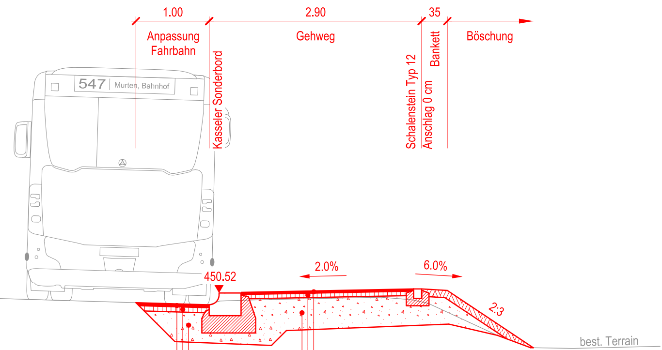
Normalprofil 1 : 50
